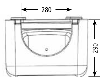
Armoire intérieure PPE vue du haut (Art. 35248).
