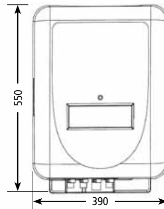
Armoire intérieure PPE vue de face (Art. 35248).
