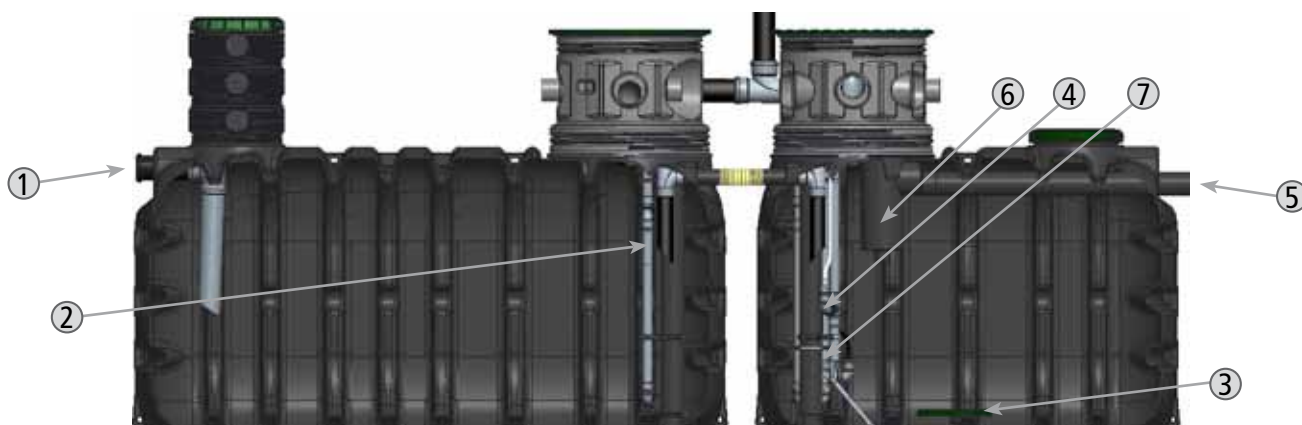
Vue de coupe d'une micro-station ACTIBLOC® 6EH (3500-2500 SL).
