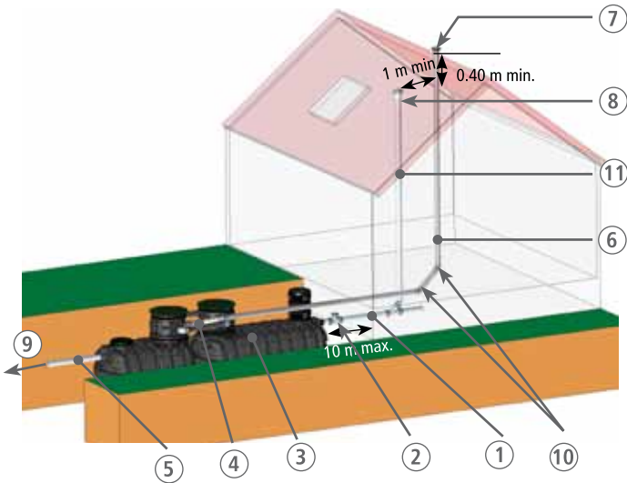
Schéma de raccordement de la ventilation haute pour une micro-station ACTIBLOC® 6EH (3500-2500 SL).
