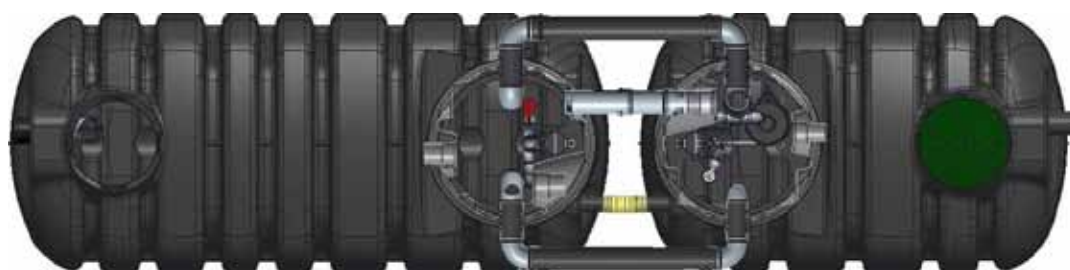
Vue de coupe d'une micro-station ACTIBLOC® 6EH (3500-2500 SL).
